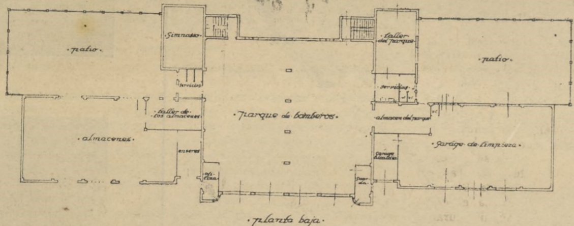
Proyecto de Parque de Bomberos, garages y almacenes municipales. Escala 1:100.
