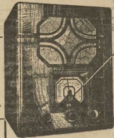
521 A.—SUPER-OCTODO. corriente alterna, ondas cortas y largas. 521 U.—Iguel modelo, para corriente continua y alterna, indistintamente.
