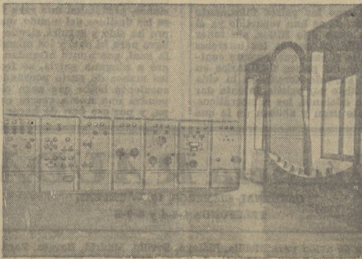
El aspecto exterior del transmisor Telefunken en la Ciudad Vaticana, se distingue por la claridad de su disposición y su sencillez. A la derecha, la instalación de conmutación para las distintas antenas dirigidas
