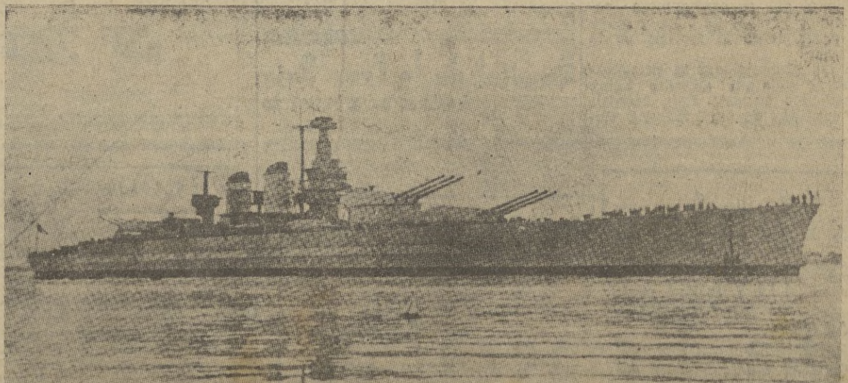
El acorazado italiano "Vittorio Veneto", la más moderna nave de guerra del mundo, de 35.000 toneladas, con una potencia de 130.000 caballos y la velocidad de 30 nudos por hora, que ha superado recientemente la prueba de máquina.
