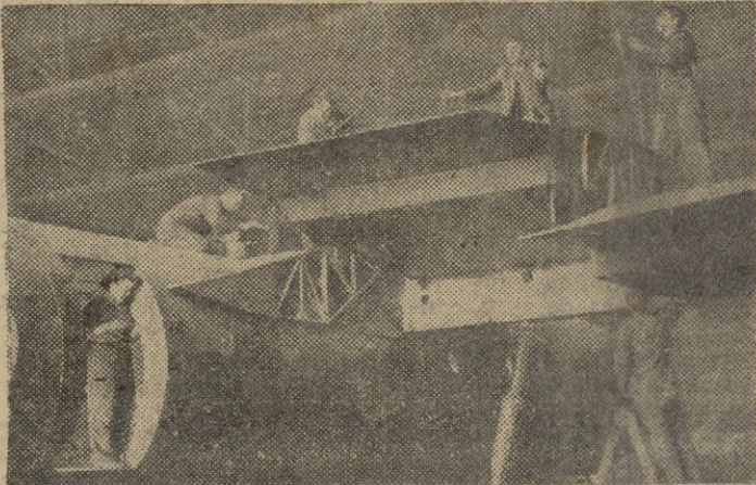
Construcción del "Horsa", el gigantesco planeador de transporte.
