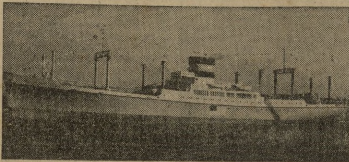
Un barco mercante americano del nuevo tipo C-3; tiene mayor capacidad de carga y mayor velocidad que el C-2. Tiene alojamiento para 12 pasajeros, 47 oficiales y tripulación. Estos barcos tienen 7.886 toneladas y una capacidad de carga de 10.026 toneladas. Velocidad normal, 16 nudos y medio.
