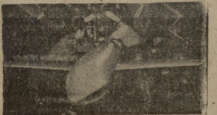
Lanzado por un avión «mosquito» de la RAF a más de 11 kilómetros de altura sobre el Atlántico, el aparato-cohete supersonico Vickers, controlado por radio, voló unos 90 segundos antes de sumergirse en el mar. En la foto colócan el aparato-cohete en el «mosquito» de la RAF.—(Calpe)
