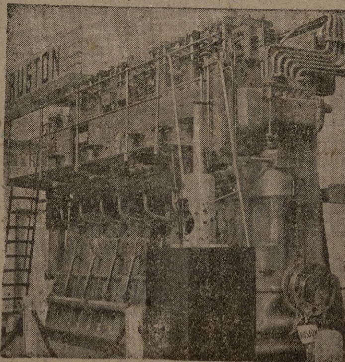
En una reciente exposición de ingeniería celebrada en Londres figuraba este potente motor marino que tiene un peso de 50 toneladas.—(Calpe)
