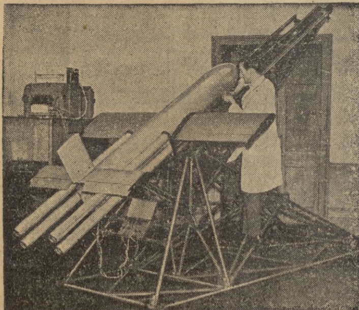
El primer proyectil británico controlado por radio, sobre el que se ha estado trabajando en secreto durante 18 meses, ha realizado con éxito una serie de vuelos de prueba. Desde tierra se ejerce un control absoluto del proyectil en pleno vuelo. --(Galpe).
