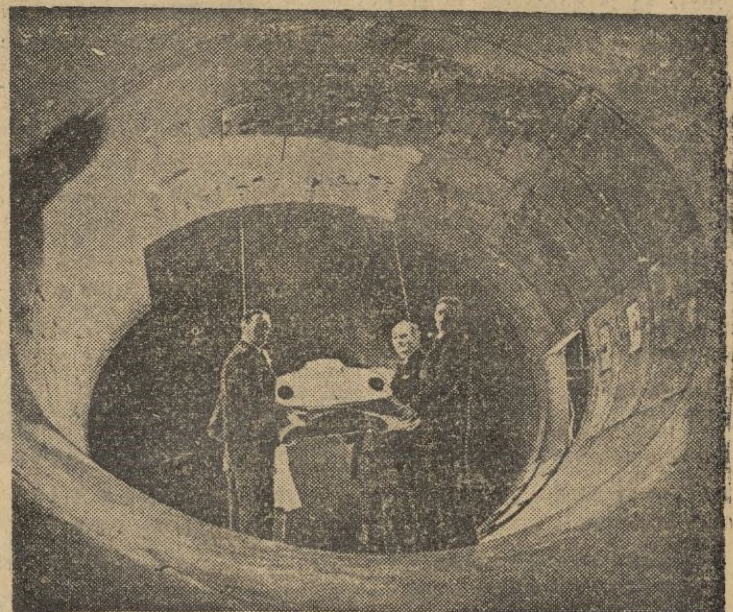
La canoa «Pájaro Azul» con su motor de reacción de 5.000 h. p. está a punto de terminarse en Pirtsmoutr, y se cree que alcanzará la velocidad de 170 millas por hora. La fotografía nos muestra a Sir Malcolm Campbell y al Jefe de Aerodinámica de la Fairey Aviation Company con el modelo de la canoa «Pájaro Azul», en el túnel aerodinámico. (Galpe)
