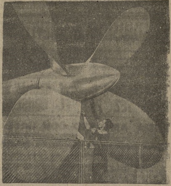
Hélice de ocho toneladas construida en Inglaterra, para un buque noruego de 16.000 toneladas de desplazamiento. Esta hélice hace 123 revoluciones por minuto. —(Galpe).
