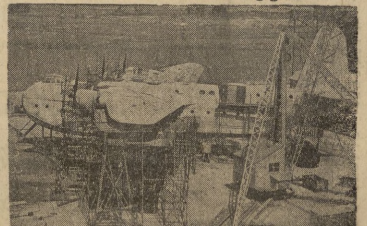
A orillas del río Medway se construye el gigantesco avión británico “Short-Sarc-Shetland”. El procedimiento de fabricación, como se ve no difiere mucho de un trasatlántico.—(Calpe).
