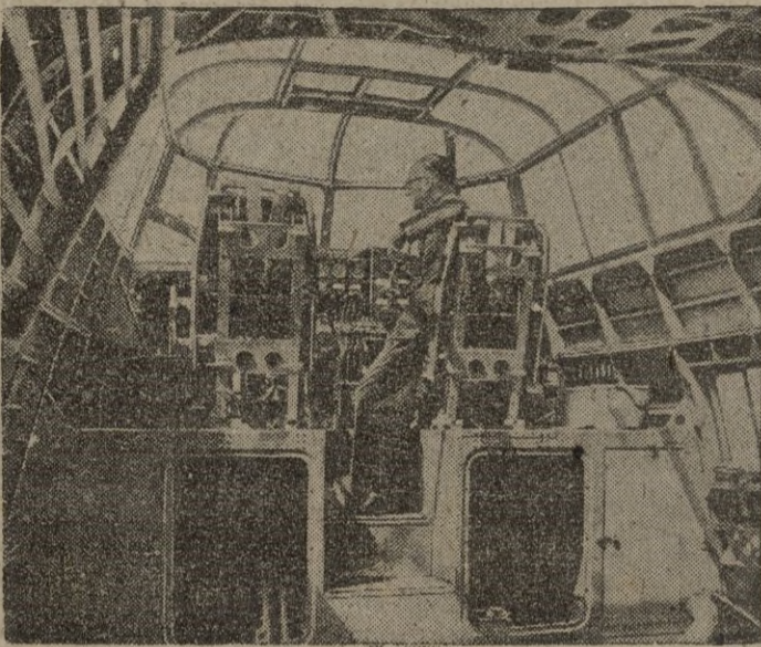
El "Short-Saro Shetland", con 70 pasajeros y 11 tripulantes, surcará los aires a fines de mes. Una idea de la magnitud del nuevo titán del espacio, construido en la Gran Bretaña, nos la da el aspecto de la carlinga del avión.— (Calpe)
