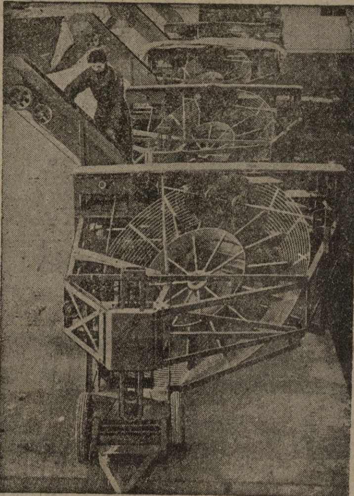
Nueva máquina industrial para productos agrícolas. Hace el trabajo de 20 obreros. Para su manejo se necesitan tres operarios y su rendimiento alcanza a 60 toneladas en 8 horas. En la foto, varias máquinas dispuestas para su embalaje.
