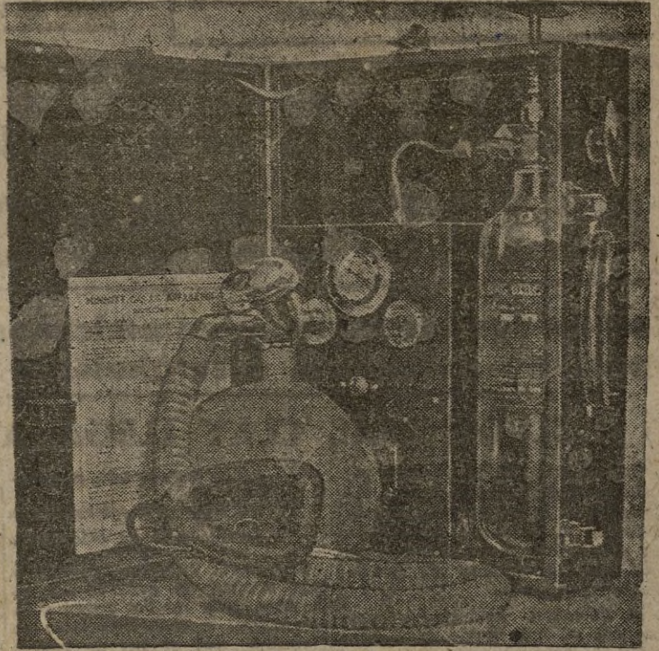
Aparato portátil para analgesia, presentado en una exposición de material y equipo para hospitales, en Londres. Pesa menos de ocho kilos y sus reducidas dimensiones le hacen muy apropiado para el manejo por el propio enfermo, quien por su respiración regula la corriente de gas y aire.—(Calpe)
