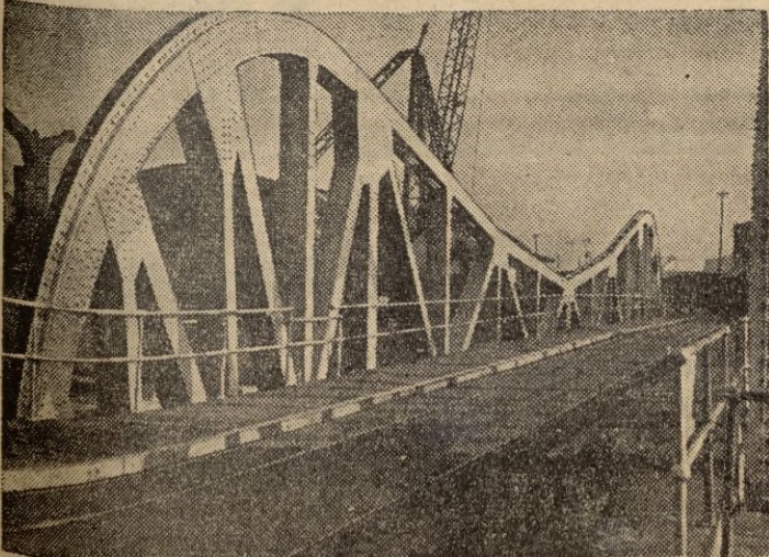
Fotografía del primer puente de aluminio del mundo. Su construcción ha costado 85.000 libras esterlinas. No pesa más de 54 toneladas y su longitud es de 27.50 metro. Admite tráfico ferroviario y de carretera.
