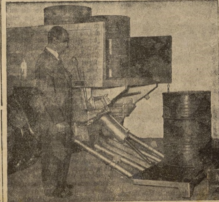
Cargador mecánico para camiones. Lo maneja un solo obrero y, una vez cargado el vehículo, cierra la parte posterior de éste. Puede admitir pesos de 700 kgs.
