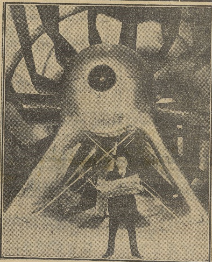
Esta espectacular y extraña fotografía corresponde a un túnel aerodinámico para probar los motores de la National Advisory For Aeronautic. El Dr. Dryden, presidente de la Compañía aparece a la entrada del túnel.
