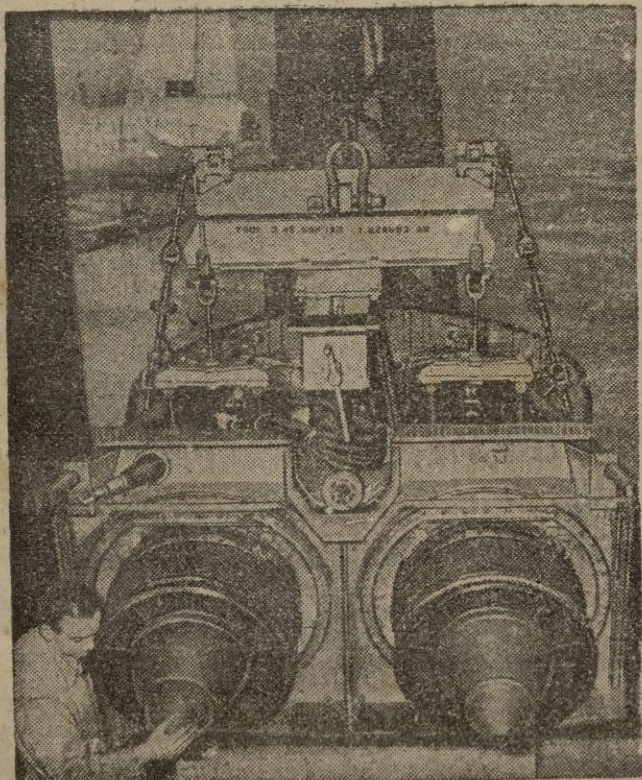
Colocación de los dos primeros motores en el hidroavión de 140 toneladas, actualmente en construcción en la isla de Wighth, que irá provisto de diez motores Bristol "Proteus".— (Foto Calpe.)
