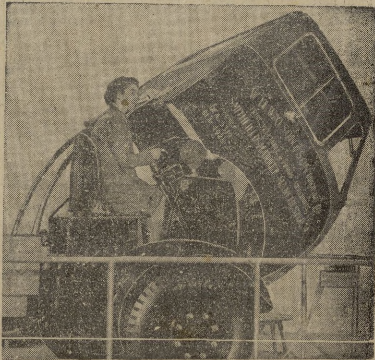
En la feria de la Gran Bretaña se ha exhibido este original modelo de camión que se desmonta con la misma facilidad con que uno se quita el sombrero. Así queda el motor completamente al descubierto.
